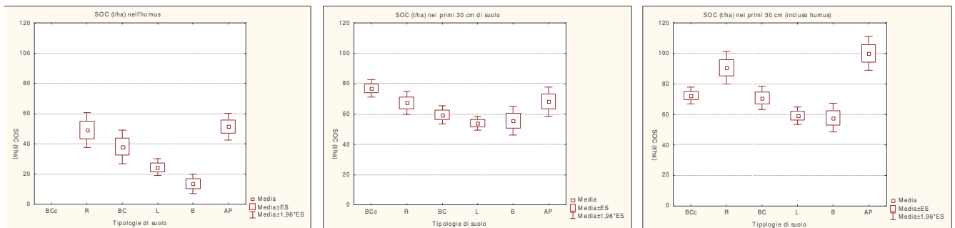
Figura 9. Stock di carbonio organico (t/ha) nell'humus, nei primi 30 cm di suolo e nei primi 30 cm di suolo includendo l'humus, nei diversi tipi di suolo della montagna del Veneto.
