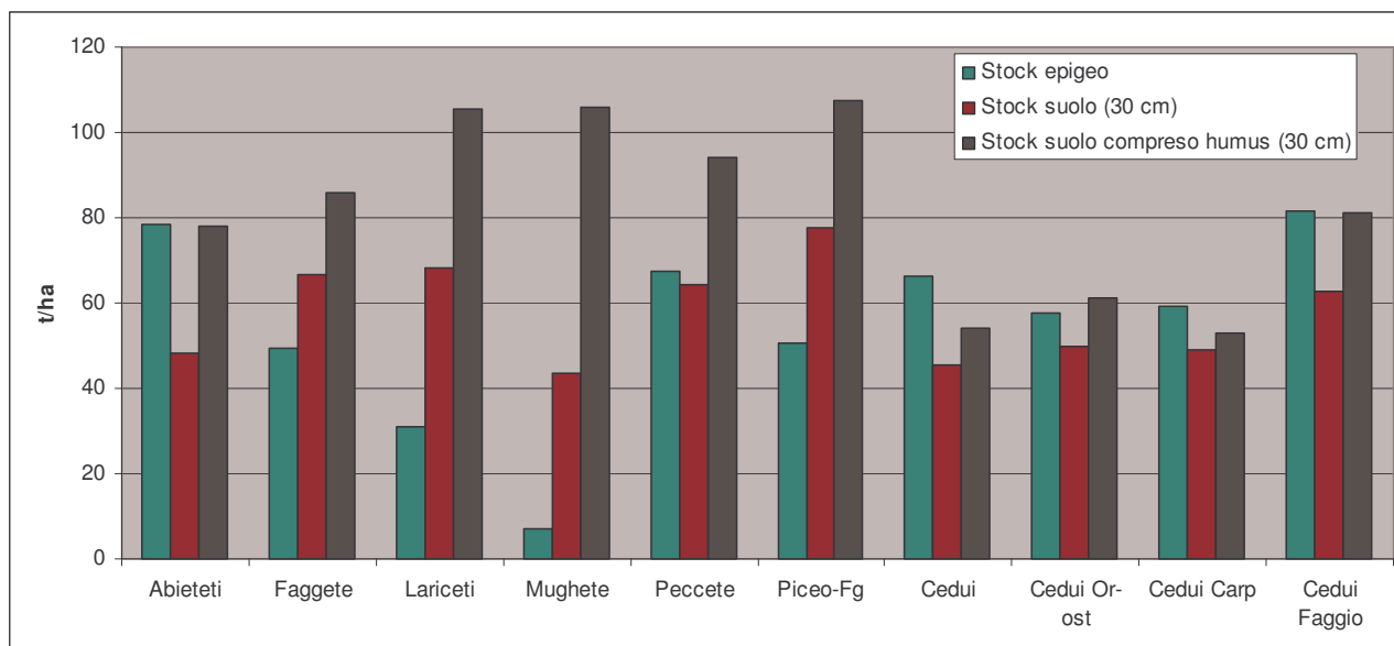
Fig. 8 - Stock di carbonio organico nella porzione epigea, nei primi 30 cm di suolo minerale e nei primi 30 cm includendo gli orizzonti organici (t/ha) nelle diverse tipologie forestali del Veneto (per lo stock di carbonio epigeo, fonte: Anfodillo et al. , 2006).
