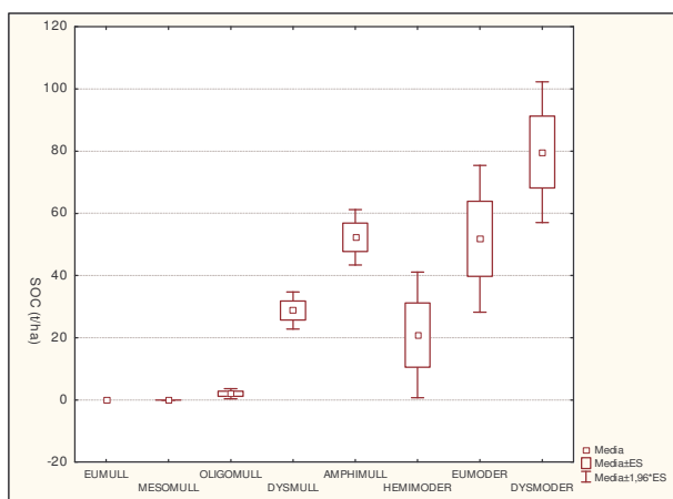
Fig. 2 - Stock di carbonio (t/ha) negli orizzonti organici delle diverse classi tassonomiche di humus (AFES, 1995).
