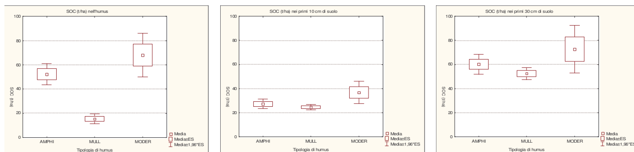
Fig. 1. - Box & whisker plots dello stock di carbonio (t/ha) nell'humus, nei primi 10 cm di suolo minerale, e nei primi 30 cm di suolo minerale, per le diverse tipologie di humus (Jabiol et al., 2004).
