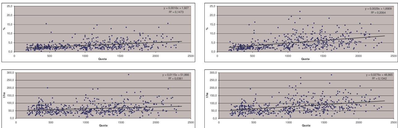
Fig. 5 - Relazione tra quota e carbonio organico (%) nei primi 30 cm di suolo (in alto a sx) e includendo gli orizzonti organici (in alto a dx), e relazione tra quota e SOC (t/ha) nei primi 30 cm di suolo minerale (in basso a sx) e includendo gli orizzonti organici (in basso a dx). Fig. 5 – Relationship between altitude and organic carbon content (%) in 0-30 cm mineral soil (top left) and in the same layer including organic horizons (top right); relationship between altitude and SOC (t/ha) in 0-30 cm layer of mineral soil (bottom left) and including organic horizons (bottom right).
