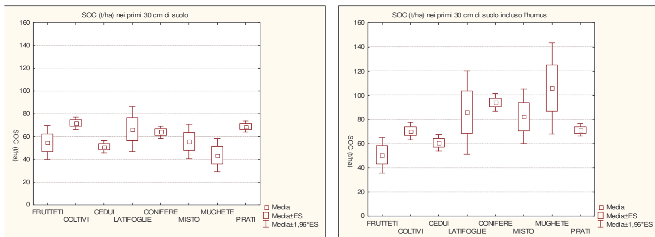
Fig. 7 - Stock di carbonio organico nei primi 30 cm di suolo minerale (a sx) o includendo gli orizzonti organici (a dx) in base al diverso uso del suolo.
