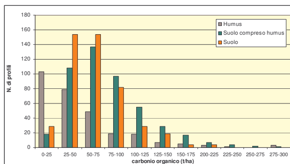
Fig. 3 - Istogramma di frequenza del contenuto medio in carbonio organico (%) e dello stock (t/ha) nell'humus, nei primi 30 cm di profondità di suolo minerale (min) e in ambedue (humus + min).
