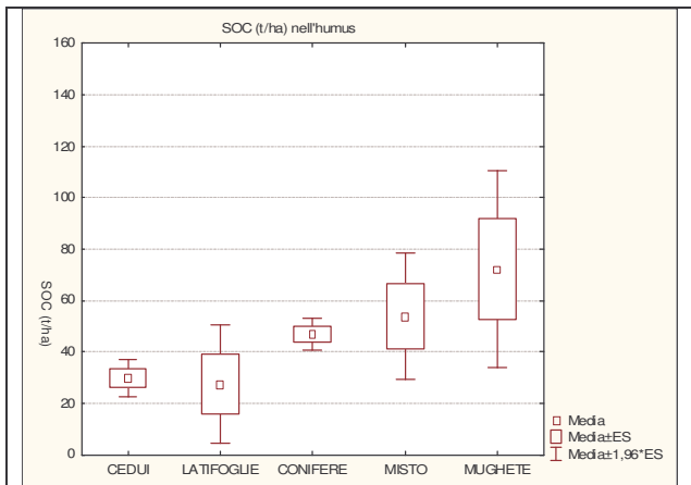
Fig. 6 - Stock di carbonio organico (t/ha) nell'humus nelle diverse formazioni forestali del Veneto.
