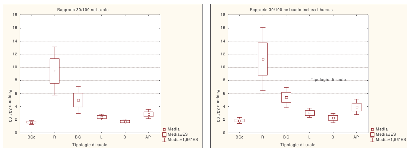
Fig. 10 - Rapporto tra stock di carbonio organico nei primi 30 cm e quello presente tra 30 e 100 cm, nel suolo (sx), e includendo l'humus (dx), per i diversi tipi di suolo della montagna del Veneto.
