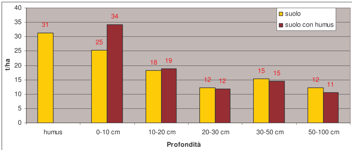
Fig. 4 – Andamento con la profondità dello stock di carbonio (mediane), includendo o meno gli orizzonti organici. Fig. 4 – Organic carbon trend with depth (median), with and without organic horizons contribution.
